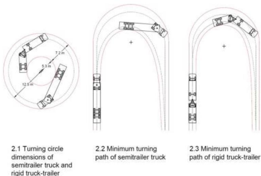
Figura 3.2 Raza de curbura a diferitelor tipuri de camioane pentru transportul animalelor. 2.1 Dimensiunile de întoarcere a camionului cu semiremorcă și a ansamblului rigid remorcă-cap tractor. 2.3. Ruta minimă de întoarcere a camionului cu semiremorcă. 2.3. Ruta minimă de întoarcere a ansamblului rigid remorcă-cap tractor.
