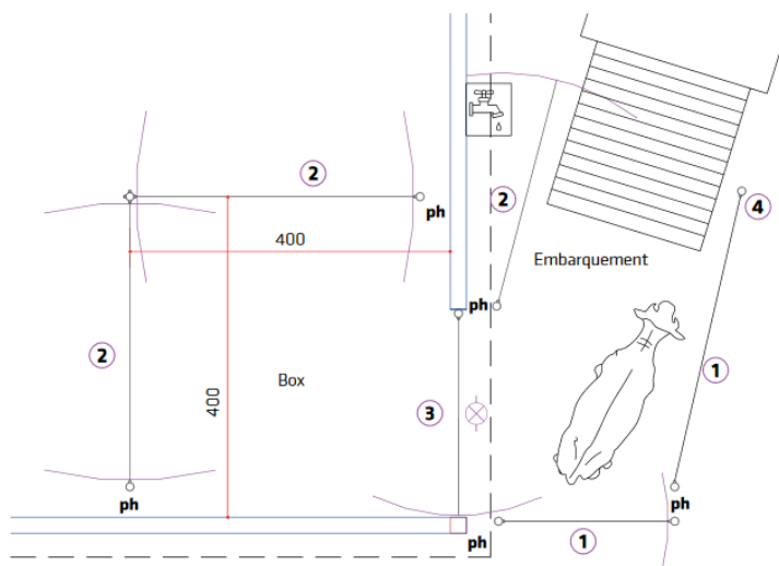
Figura 2.3 Exemple de dimensiuni adecvate ale zonei de încărcare.
