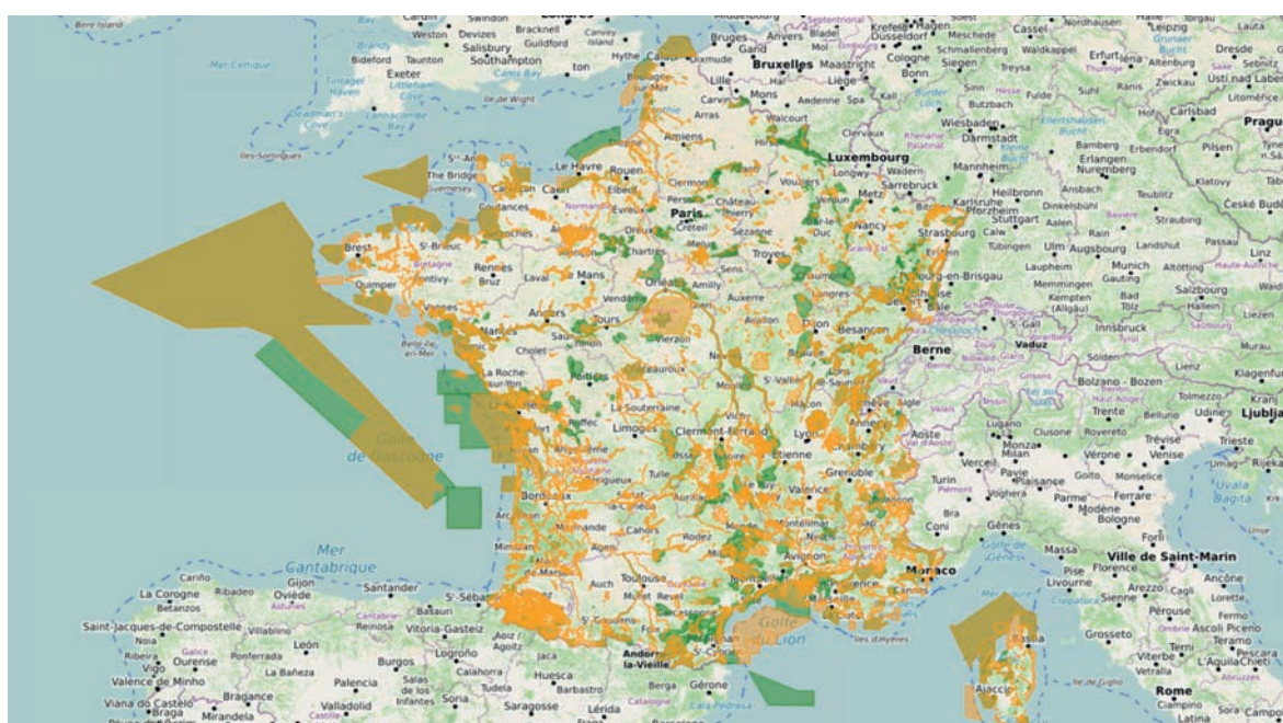
Carte des sites Natura 2000 français classés au titre de la Directive Habitats (jaune) et au titre de la Directive Oiseaux (vert). Source : MapGeoData
